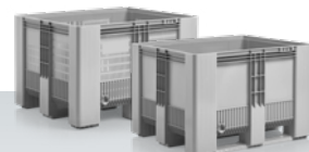
SB3 610 I Spód na 3 płozach lub 9 stopach Pełne lub perforowane ściany / dno 1200 × 1000 × 790 mm Standardowe kolory:
