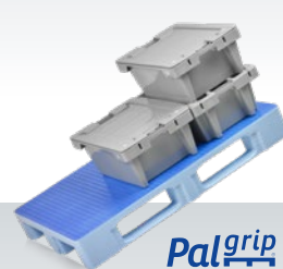
Paleta higieniczna zamknięta TC1 / TC3 / TC3-5 1200 × 800 × 160 mm / 1200 × 1000 × 160 mm
